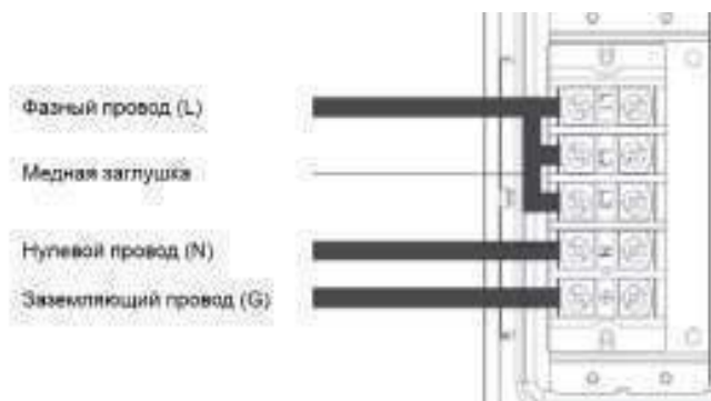
Рис. 8. Однофазное подключение прибора – зеркальный порядок
