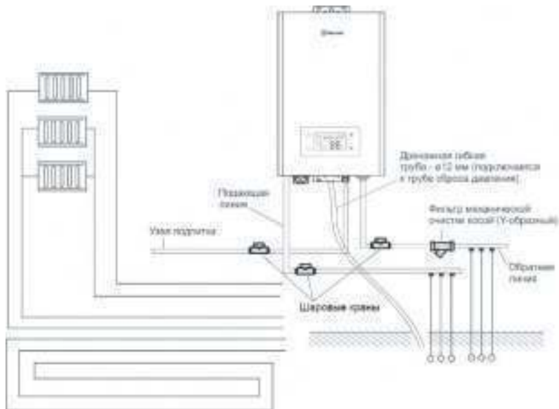
Рис. 5. Схема подключения труб
