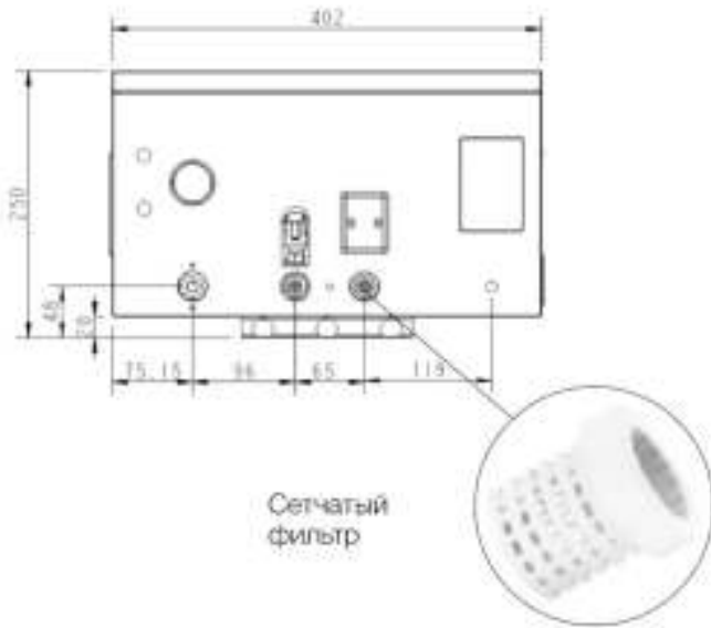
Рис. 15. Сетчатый фильтр
